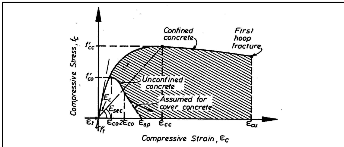
〈그림 7.2〉 Mander 등의 콘크리트 압축응력 변형률 모델
