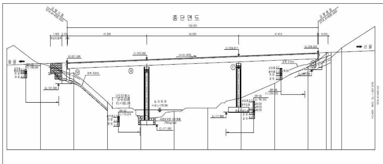
〈그림 7.5〉 물곡2교(상, 청평방향) 종단면도
