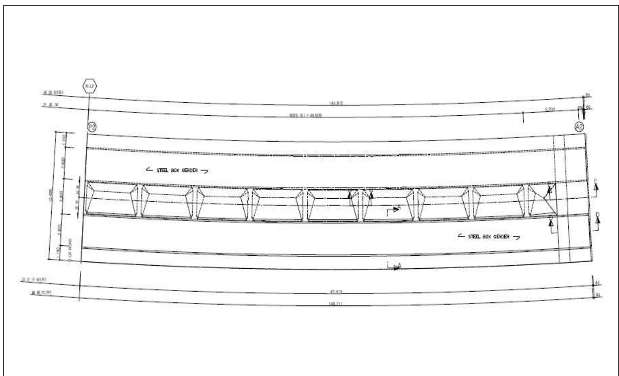
<그림 7.9> 물곡2교(상, 청평방향) 상부 일반도(3)
