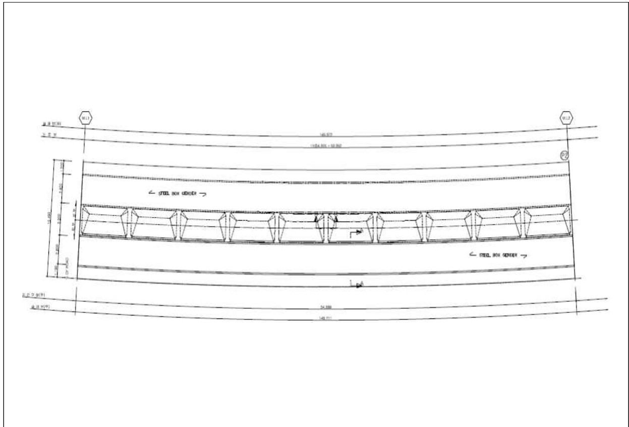
<그림 7.8> 물곡2교(상, 청평방향) 상부 일반도(2)
