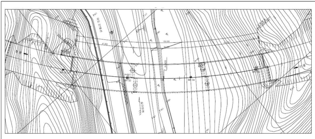
〈그림 7.4〉 물곡2교(상, 청평방향) 평면도
