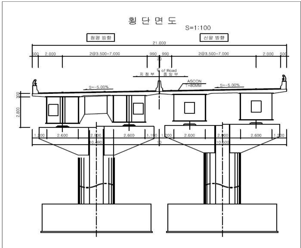
〈그림 7.6〉 물곡2교(상, 청평방향) 횡단면도
