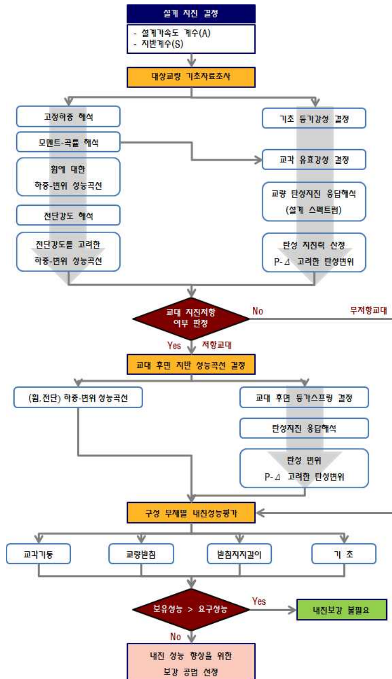
<그림 7.1> 내진성능평가 흐름도
