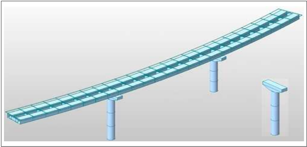
〈그림 7.12〉 물곡2교(상, 청평방향) 교량 구조해석 모델링
